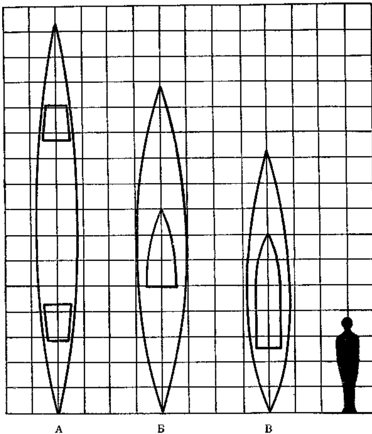
Пирого и байдарки одиночных рейсов. Сопоставление размеров: А — "Либерия II"; Б — "Немецкий спорт" Ромера; В — "Либерия III".
