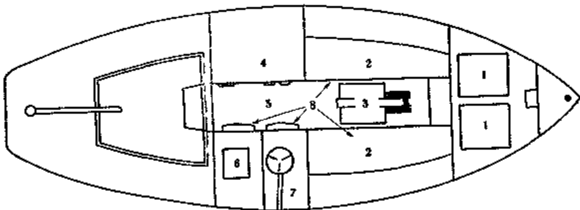
План "Нео ван". 1 — носовые люки; 2 — койки; 3 — стол; 4 — навигационный стол; 5 — кабины; 6 — умывальник; 7 — камбуз; 8 — шкафы и полки.
